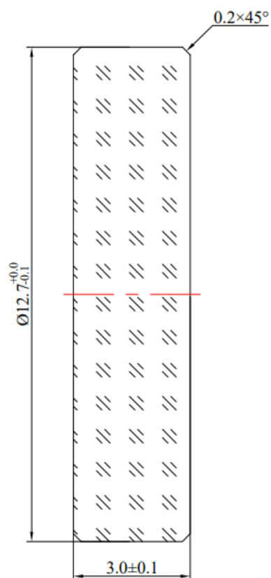
Чертеж OWB040026
