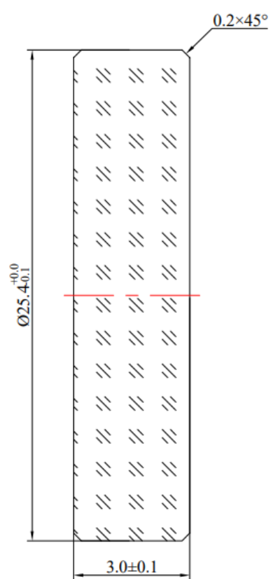
Чертеж OWB080026
